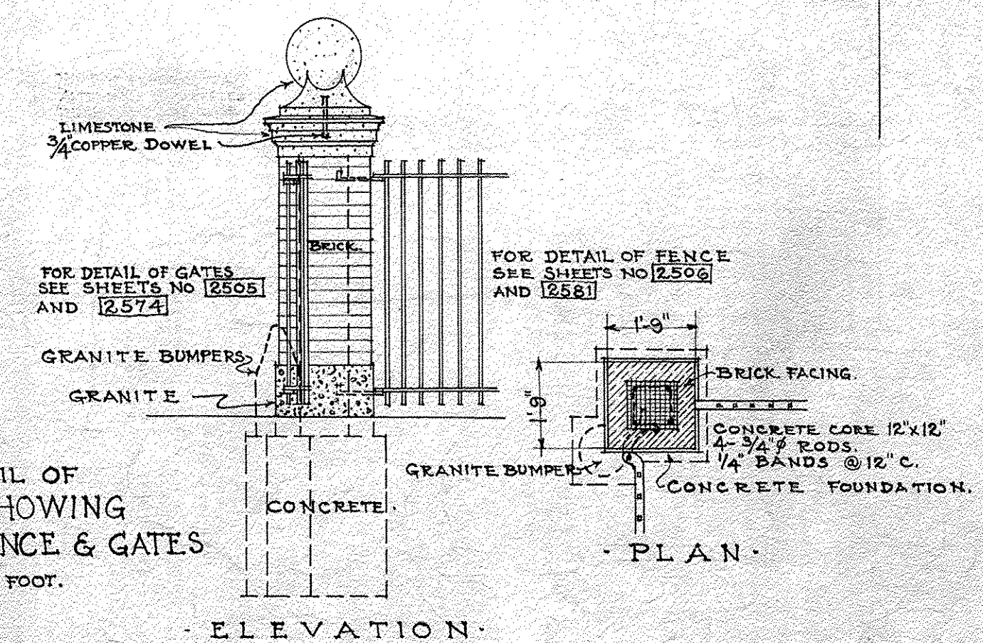
ELEVATION
